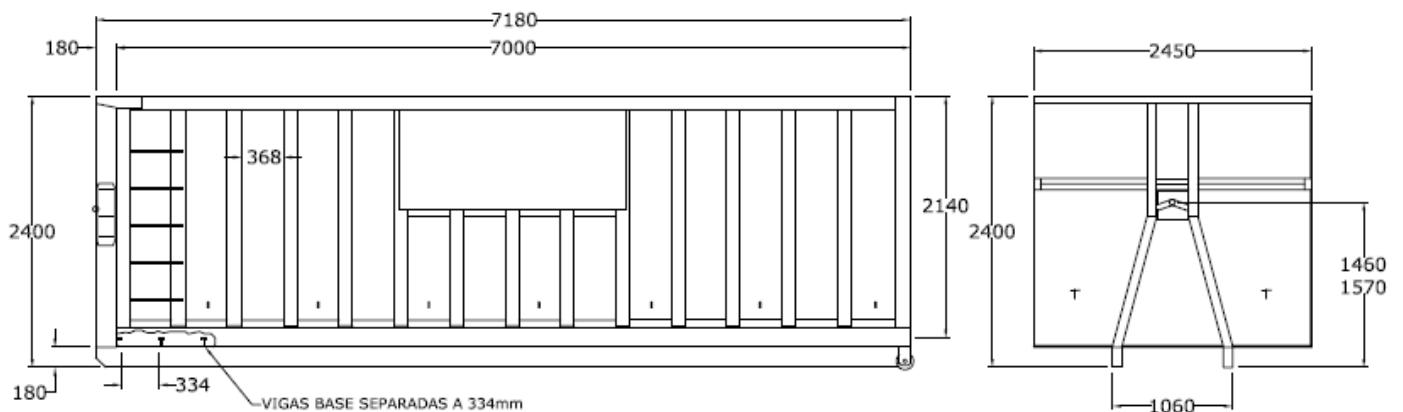
1 HOJA APERTURA BASCULANTE LATERAL
